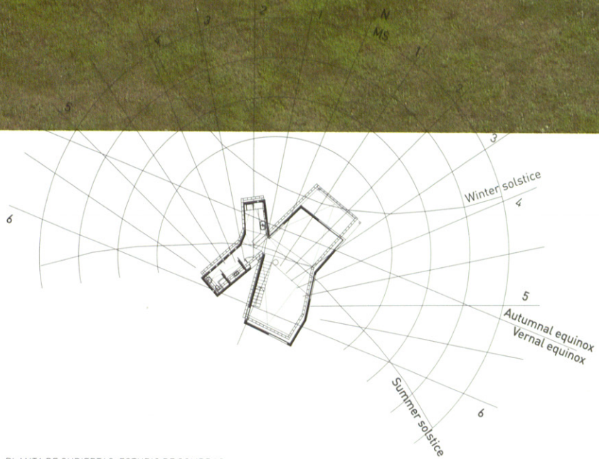
PLANTA DE CUBIERTAS, ESTUDIO DE SOMBRAS ROOF PLAN, SHADOW STUDY
